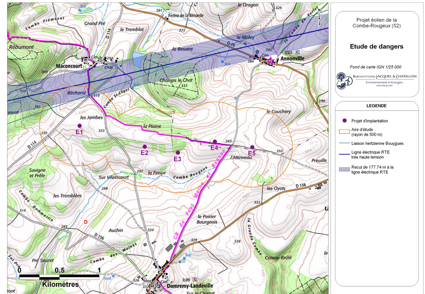
Carte 8 : Réseaux (Source : BE Jacquiel et Chatillon)
