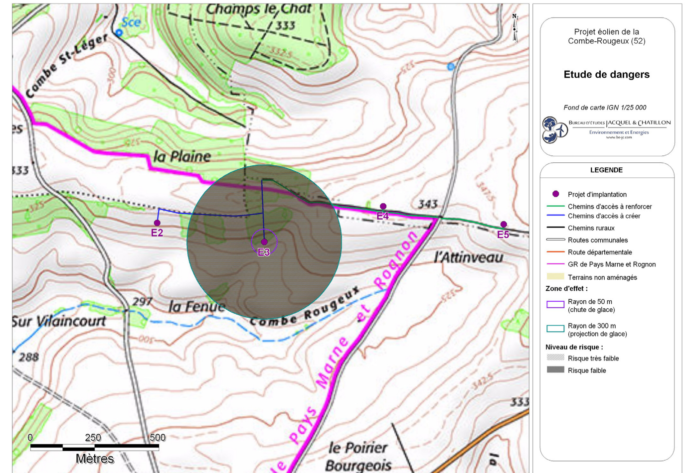
Carte 19 : Éolienne n°3 – Risques liés à la chute et à la projection de glace (Source : BE Jacquel et Chatillon)
