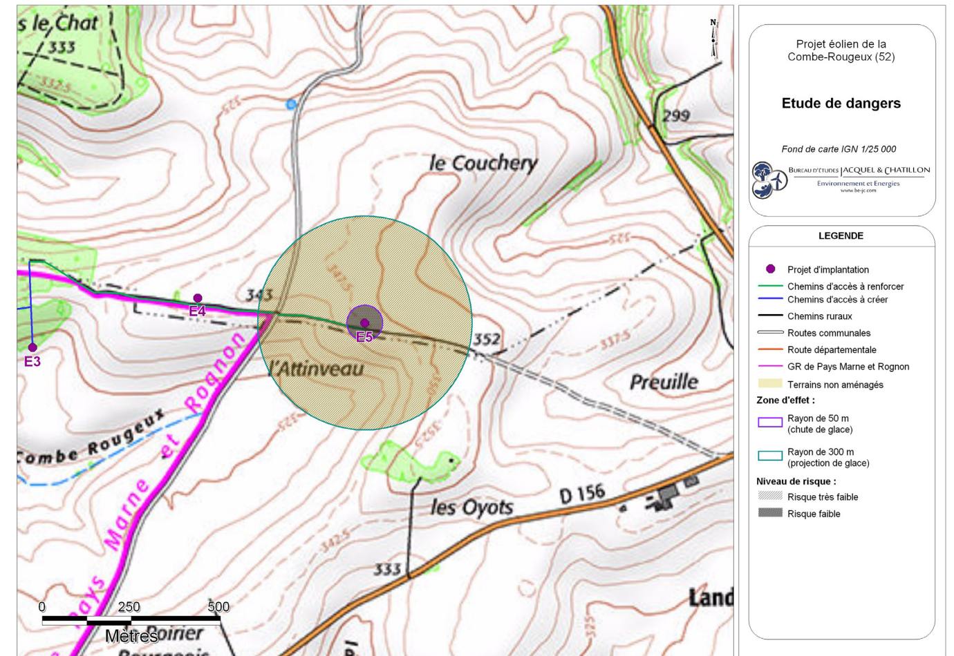
Carte 23 : Éolienne n°5 – Risques liés à la chute et à la projection de glace (Source : BE Jacquel et Chatillon)
