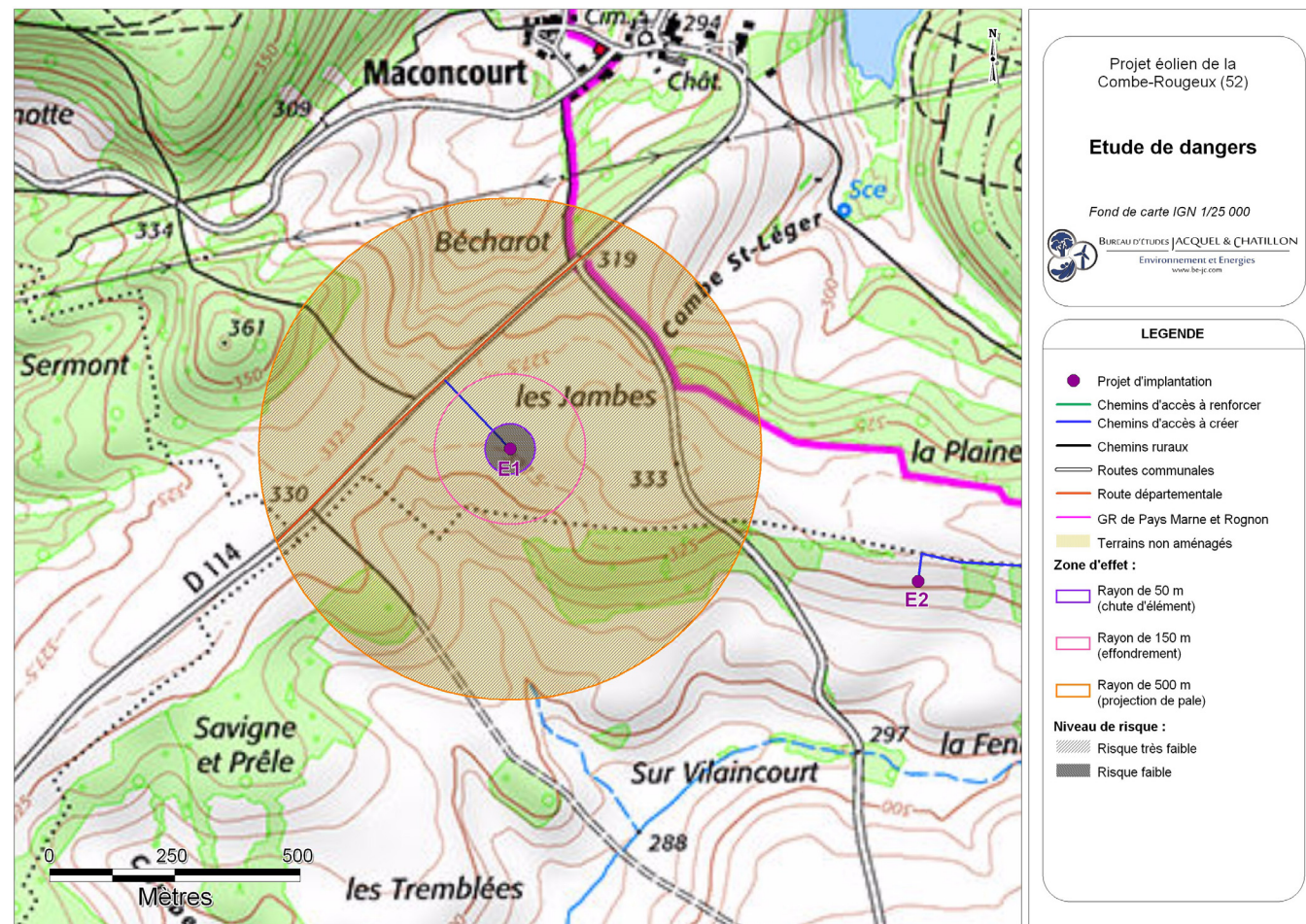
Carte 14 : Éolienne n°1 – Risques liés à l'effondrement de l'éolienne, à la chute d'élément de l'éolienne, et à la projection de pale ou de fragment de pale (Source : BE Jacquel et Chatillon)
