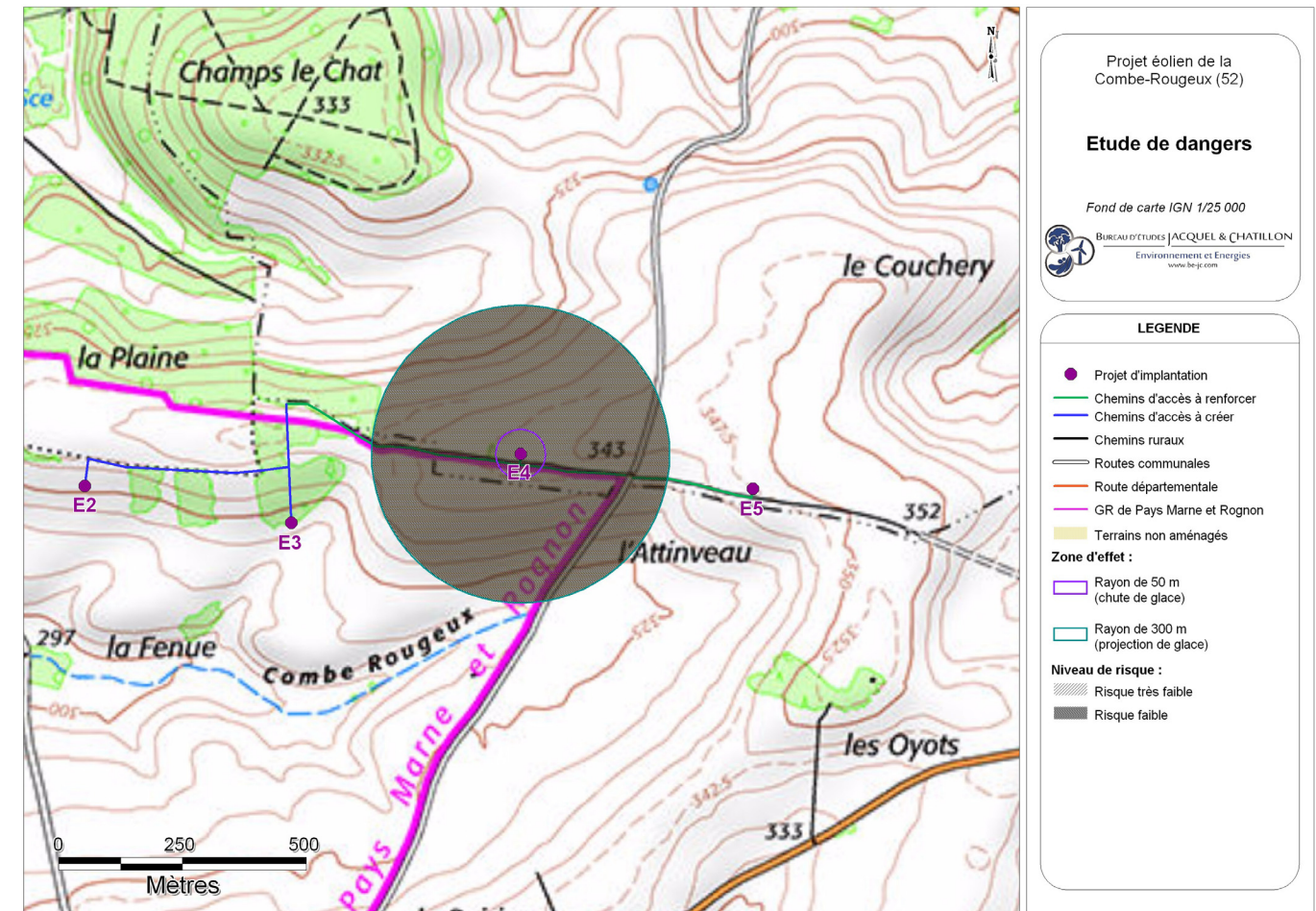
Carte 21 : Éolienne n°4 – Risques liés à la chute et à la projection de glace (Source : BE Jacquel et Chatillon)
