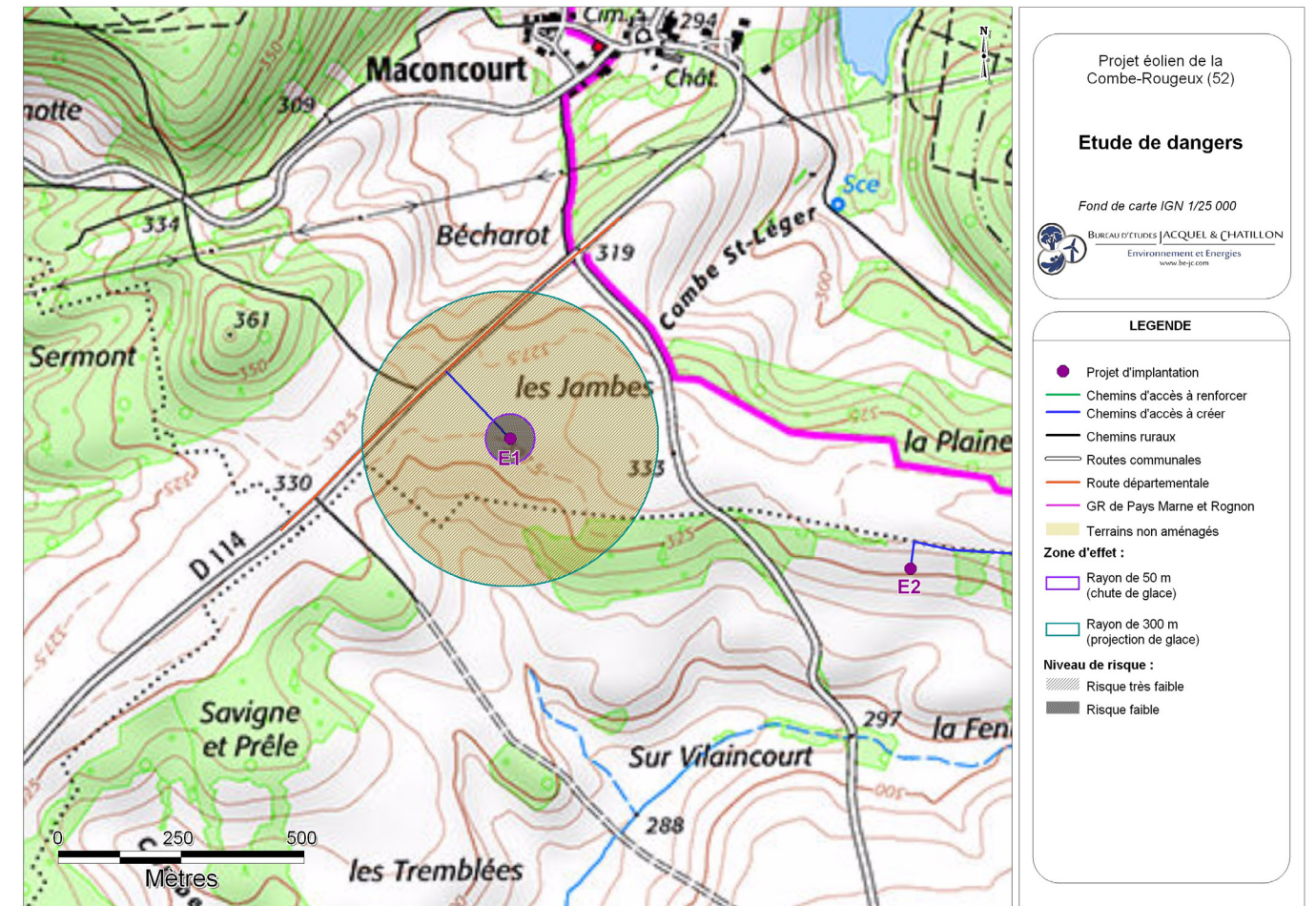
Carte 15 : Éolienne n°1 – Risques liés à la chute et à la projection de glace (Source : BE Jacquel et Chatillon)
