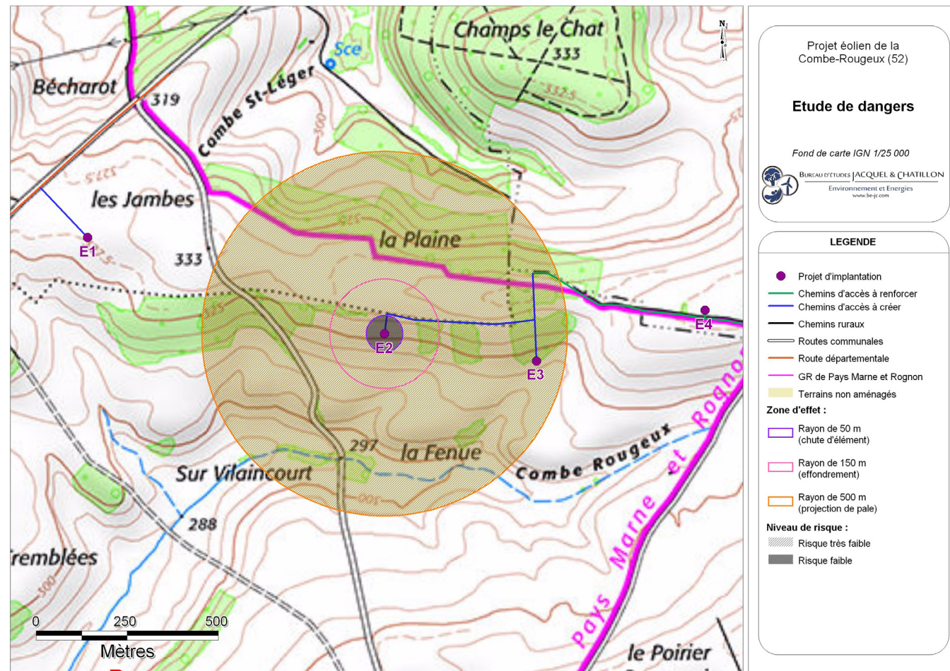
Carte 16 : Éolienne n°2 – Risques liés à l'effondrement de l'éolienne, à la chute d'élément de l'éolienne, et à la projection de pale ou de fragment de pale (Source : BE Jacquel et Chatillon)
