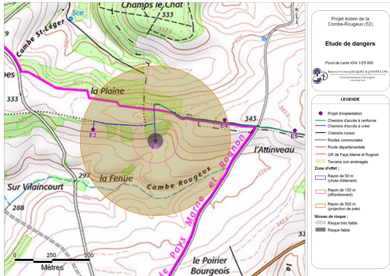
Carte 18 : Éolienne n°3 – Risques liés à l'effondrement de l'éolienne, à la chute d'élément de l'éolienne, et à la projection de pale ou de fragment de pale (Source : BE Jacquel et Chatillon)
