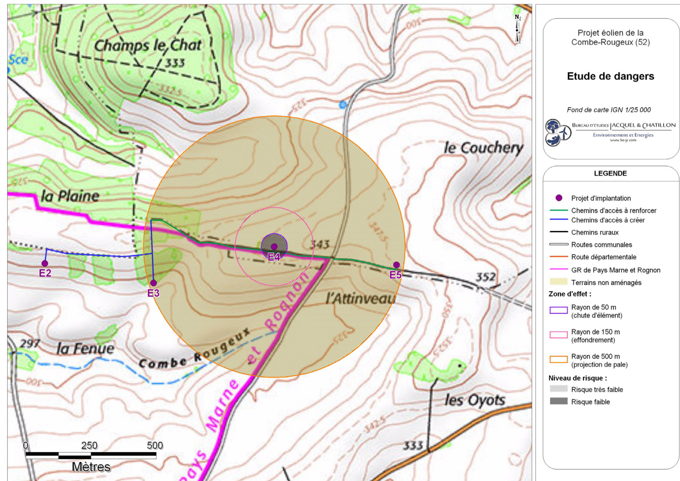
Carte 20 : Éolienne n°4 – Risques liés à l'effondrement de l'éolienne, à la chute d'élément de l'éolienne, et à la projection de pale ou de fragment de pale (Source : BE Jacquel et Chatillon)
