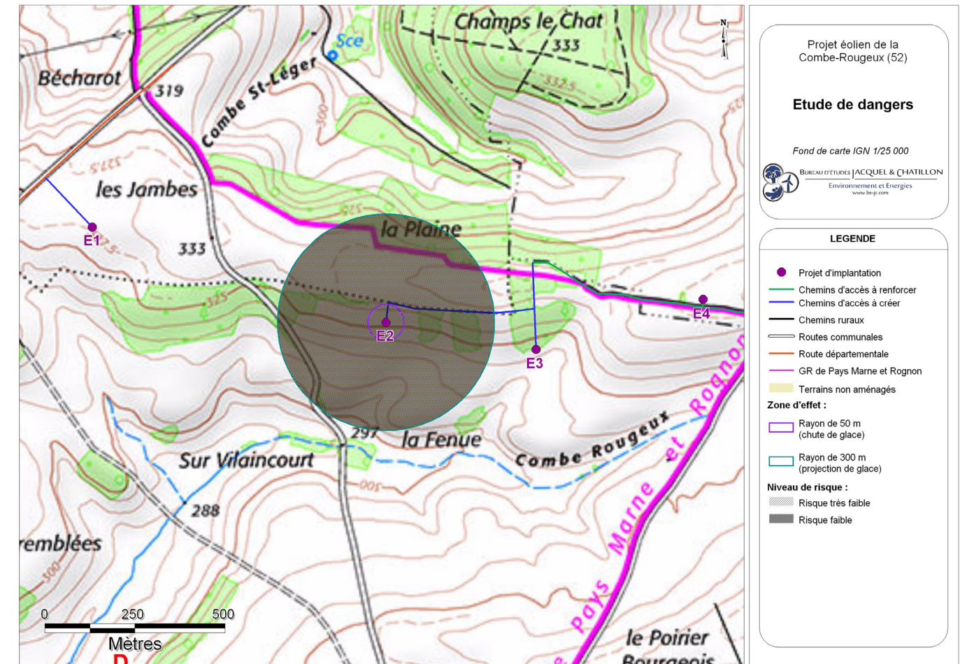
Carte 17 : Éolienne n°2 – Risques liés à la chute et à la projection de glace (Source : BE Jacquel et Chatillon)
