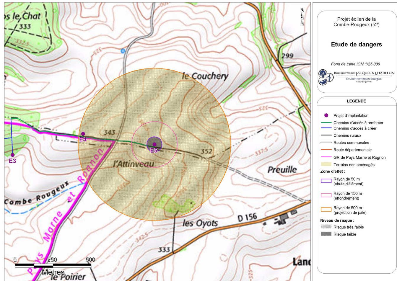
Carte 22 : Éolienne n°5 – Risques liés à l'effondrement de l'éolienne, à la chute d'élément de l'éolienne, et à la projection de pale ou de fragment de pale (Source : BE Jacquel et Chatillon)
